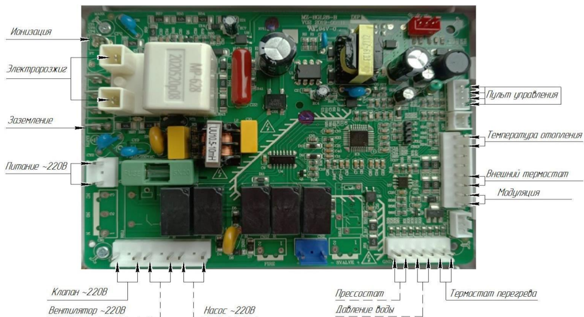
Рисунок 2 – Схема электрических подключений котла КОВ-__СТ1се
