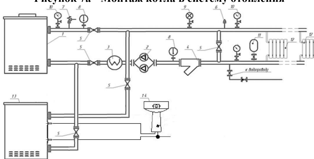
Рисунок 7а - Монтаж котла в систему отопления
